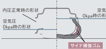
タイヤ断面図
