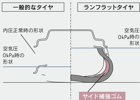
タイヤ断面図
