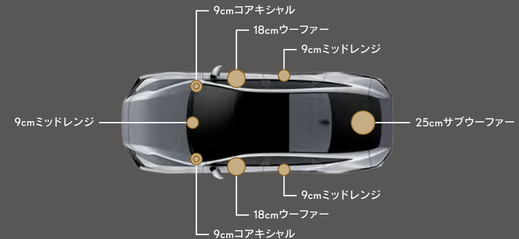
10スピーカーレイアウト
